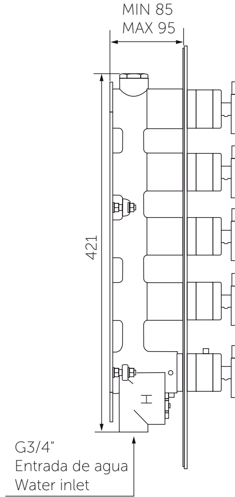
VISTA LATERAL
