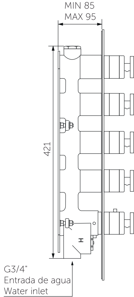
VISTA LATERAL
