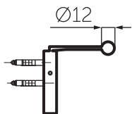
VISTA LATERAL
