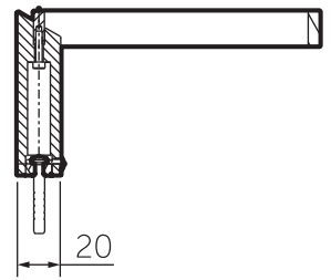
Corte A
