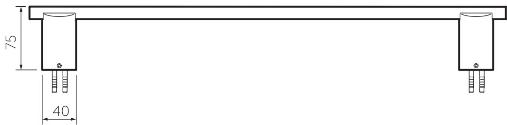
VISTA INFERIOR
