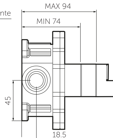
VISTA LATERAL
