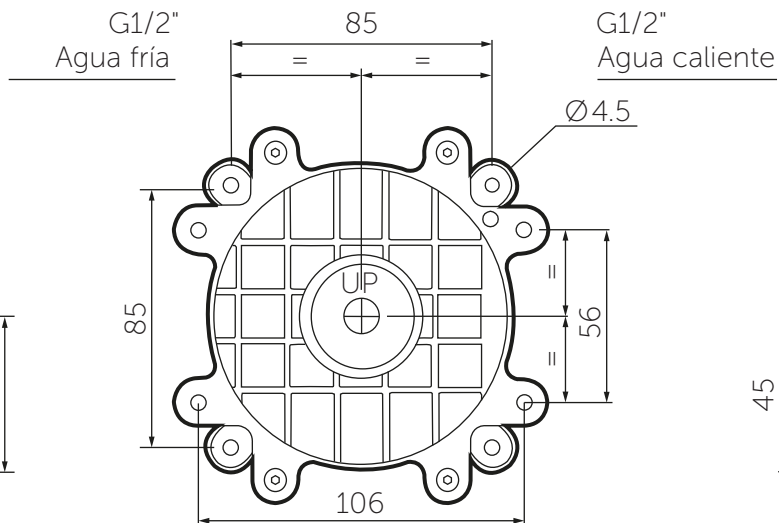
VISTA INFERIOR
