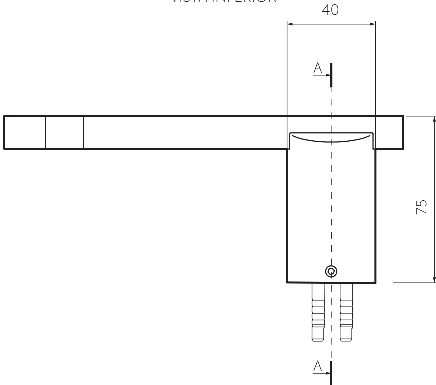
VISTA INFERIOR
