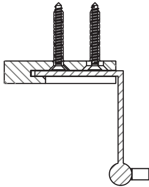
Corte A
