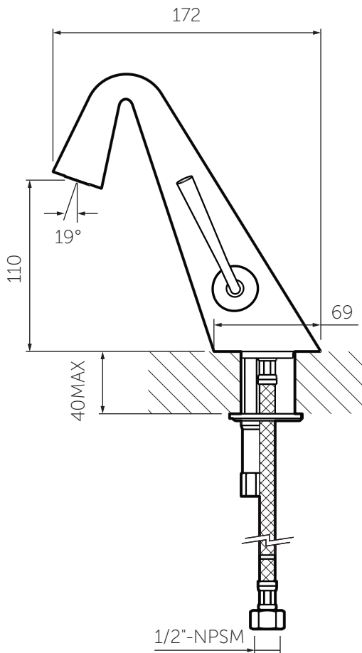
VISTA LATERAL
