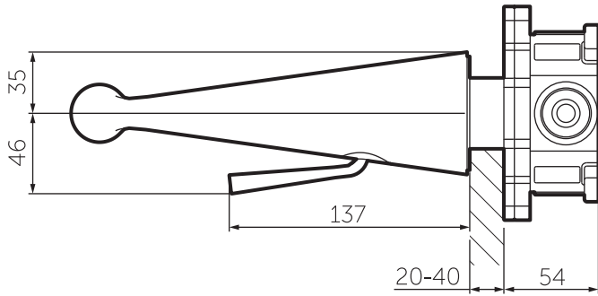
VISTA LATERAL
