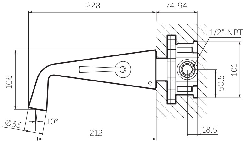
VISTA LATERAL
