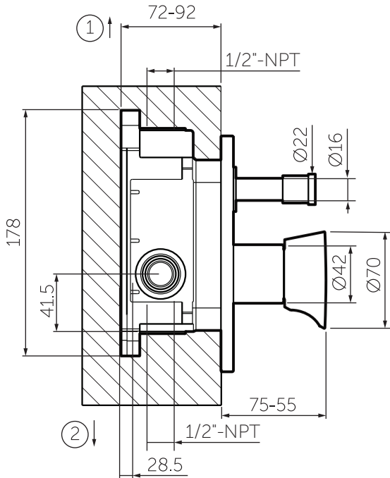
VISTA LATERAL
