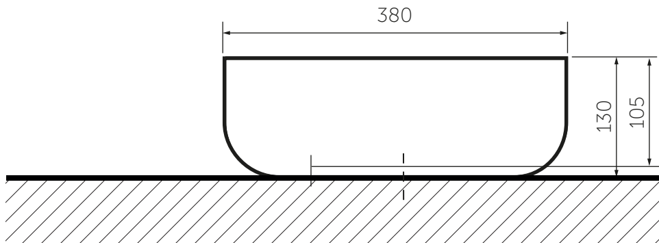
VISTA LATERAL
